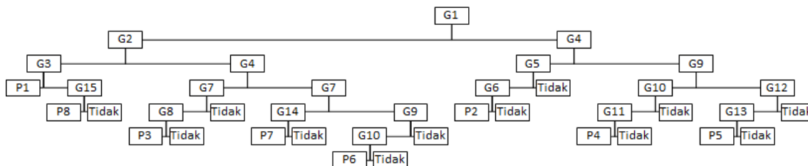
Gambar 7. Pohon keputusan
