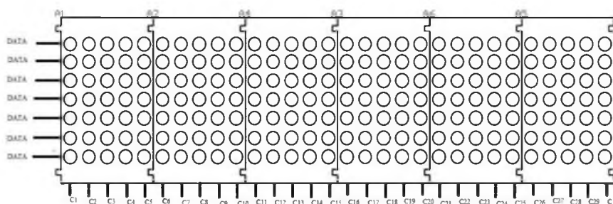
Gambar 9. Rangkaian dot matrik
