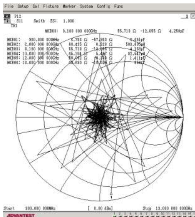
Gambar 17. Impedansi Filter
