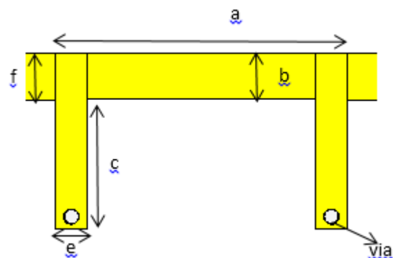
Gambar 3. Konfigurasi HPF
