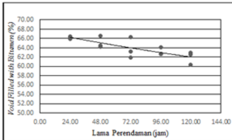
Gambar 7 Hubungan antara Lama Perendaman dengan VFB
