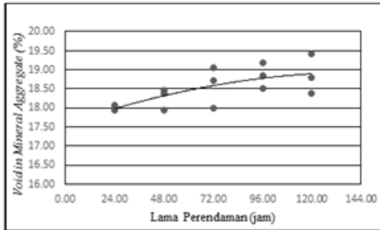
Gambar 6 Hubungan antara Lama Perendaman dengan VMA
