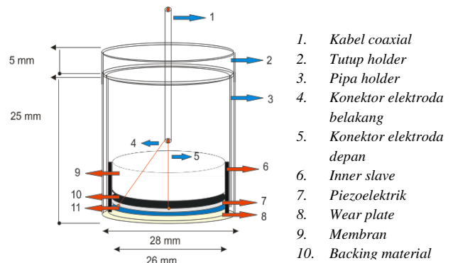
Gambar.6. Konstruksi transduser ultrasonik
