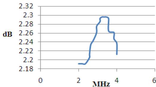
Gambar. 10. Grafik pengujian frekuensi respon secara burst.
