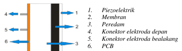
Gambar.7. Susunan backing material .
