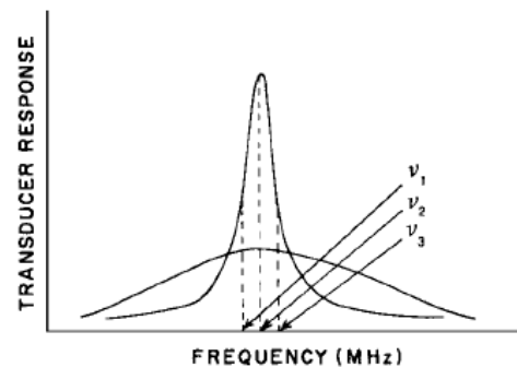
Gambar. 3. Frekuensi respon transduser ultrasonik [6]
