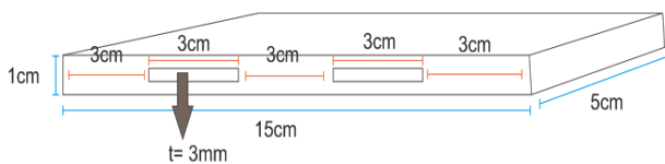
Gambar. 11. Balok uji aluminium dengan cacat.
