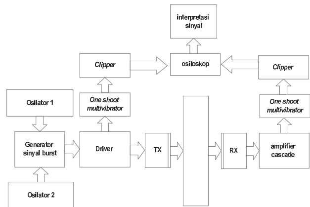
Gambar. 8. Diagram blok sistem elektronika transduser ultrasonik
