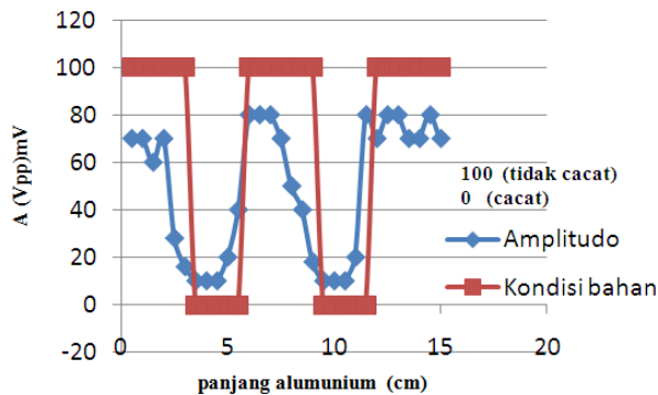
Gambar.12. Perbandingan hasil pengukuran cacat dengan kondisi bahan sebenarnya menggunakan transduser ultrasonik.
