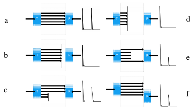
Gambar.5. Pengukuran cacat bahan padat dengan metode transmisi [10]
