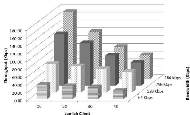
Gambar 6. Hasil Pengukuran Throughput pada saat Pengaksesan Website LSK.
