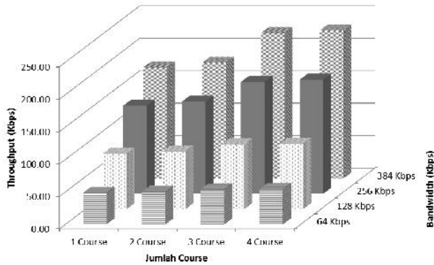
Gambar 5. Hasil Pengukuran Throughput pada sistem sinkronisasi database
