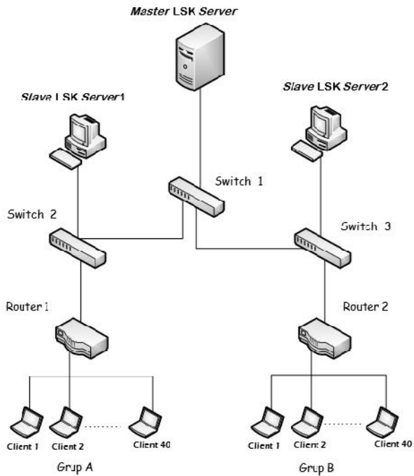
Gambar 1. Desain Topologi Jaringan
