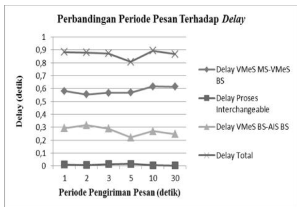
Gambar 9 Perbandingan periode pengirim pesan terhadap delay
