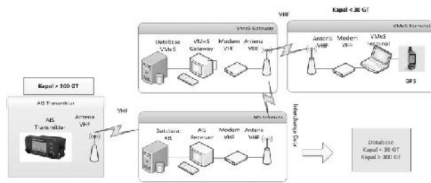
Gambar 1 Arsitektur sistem interchangeable
