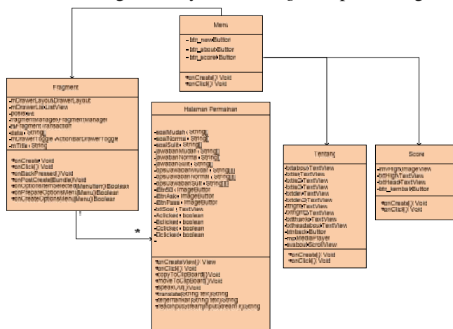
Gambar 5. Class Diagram Aplikasi Genius Quiz
