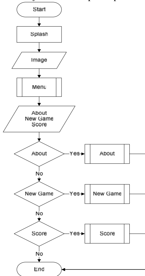
Gambar 7. Proses Perancangan Desain
