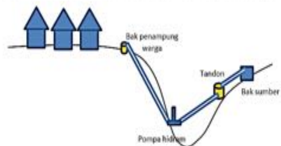
Gambar 1. Sketsa keadaan instalasi pompa hidram.
