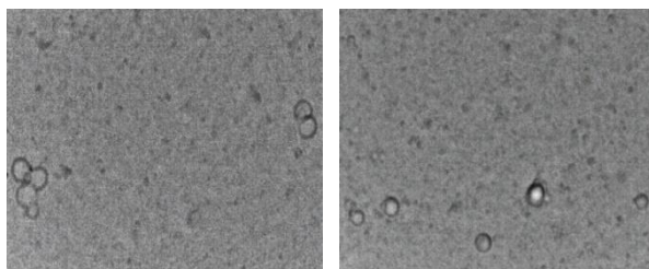
Gambar 3. Vesikel etosom pada perbesaran 1.000 kali
