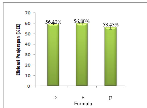
Gambar 5. Nilai Efisiensi Penjerapan Formula D: 3% fosfatidilkolin dan 30% etanol, E: 3% fosfatidilkolin dan 35% etanol, F: 3% fosfatidilkolin dan 40% etanol
