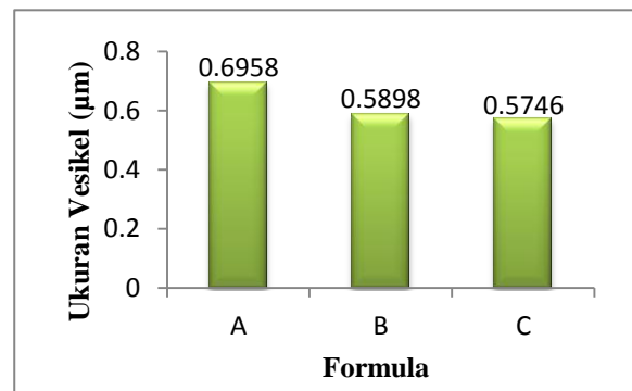
Gambar 1. Ukuran vesikel ( \mu\text{m} ) Formula A: 2% fosfatidilkolin dan 30% etanol, B : 2% fosfatidilkolin dan 35% etanol, C : 2% fosfatidilkolin dan 40% etanol.
