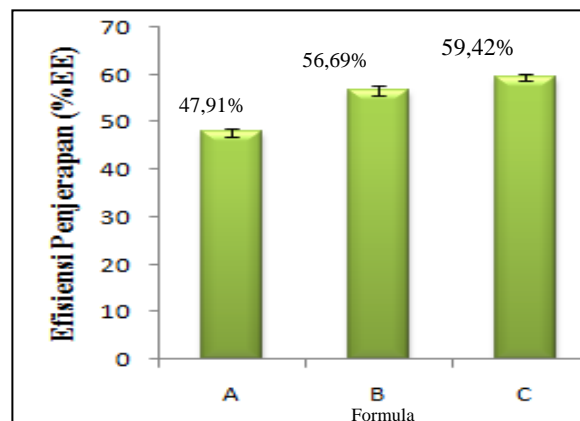
Gambar 4. Nilai Efisiensi Penjerapan Formula. A: 2% fosfatidilkolin dan 30% etanol, B: 2% fosfatidilkolin dan 35% etanol, C: 2%
