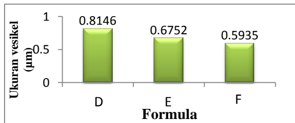
Gambar 2. Ukuran vesikel (µm) Formula D: 3% fosfatidilkolin dan 30% etanol, E : 3% fosfatidilkolin dan 35% etanol, F: 3% fosfatidilkolin dan 40% etanol
