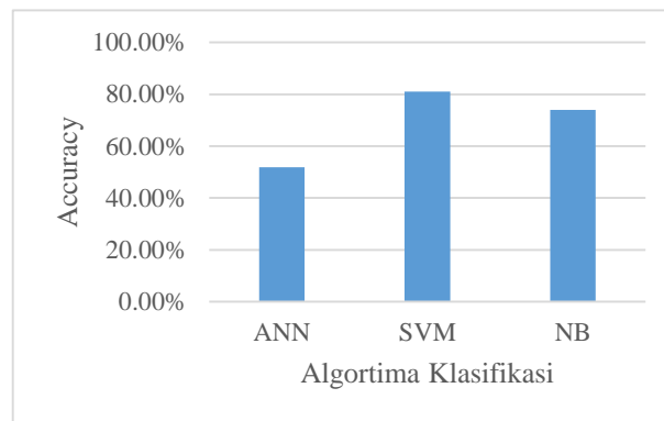
Gambar 2. Komparasi accuracy algoritma klasifikasi
