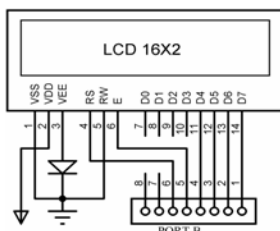
b. Rangkaian LCD 16X2
