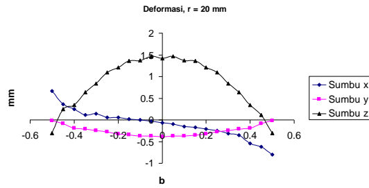
Gambar 10. Harga distribusi deformasi pada daerah antar lubang, r = 20 mm
