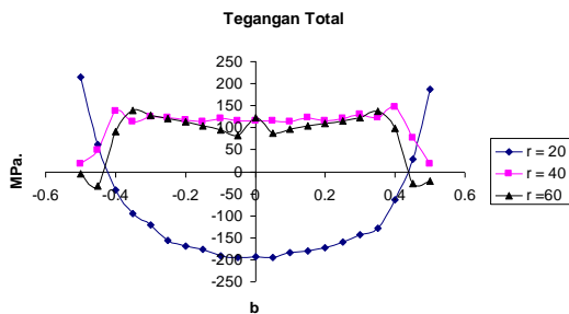
Gambar 8. Tegangan Total
