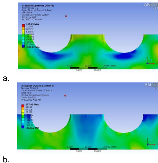
Gambar 2. Kontur distribusi tegangan normal searah sumbu x dan y
