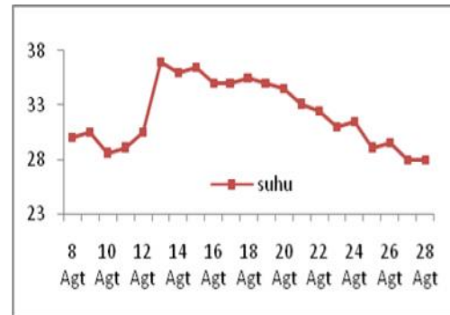
Gambar 16 – Tanpa Kontrol Suhu
