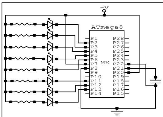
Gambar 8 – Rangkaian MK sebagai Output
