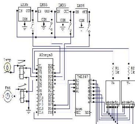
Gambar 3 – Skema Kontrol Temperatur
