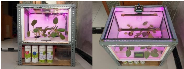
Gambar 14. Hidroponik NFT Dengan Sitem Kendali.
