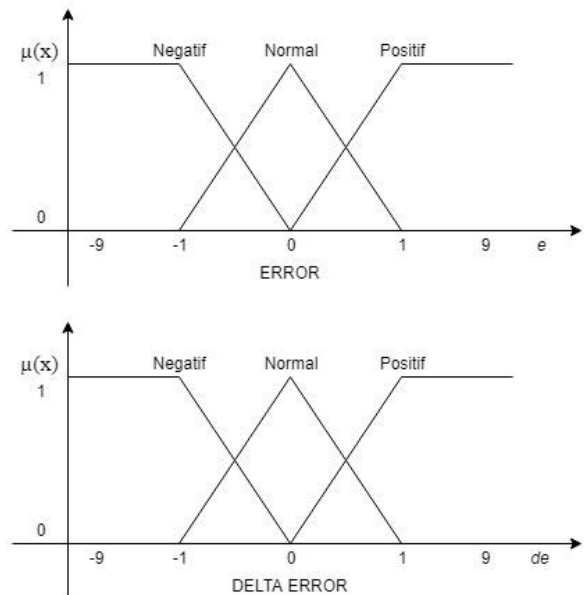
Gambar 9. Himpunan Fuzzy Error dan Delta Error Keasaman
