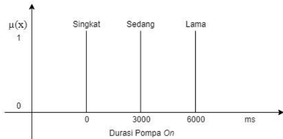
Gambar 8. Himpunan Fuzzy Durasi Pompa on Nutrisi
