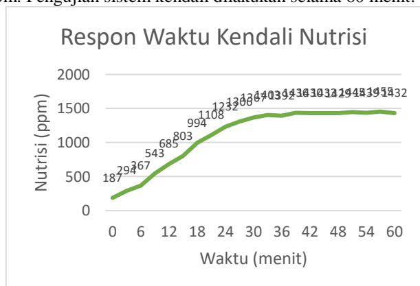
Gambar 15. Respon Waktu Kendali Nutrisi
