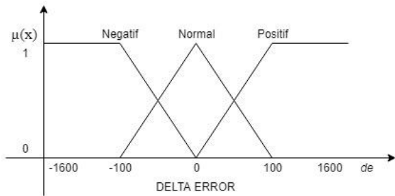
Gambar 7. Himpunan Fuzzy Error dan Delta Error Nutrisi
