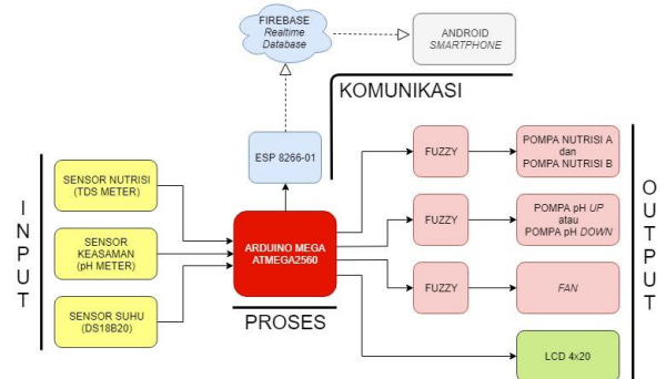
Gambar 5. Blok Diagram Sistem Alat
