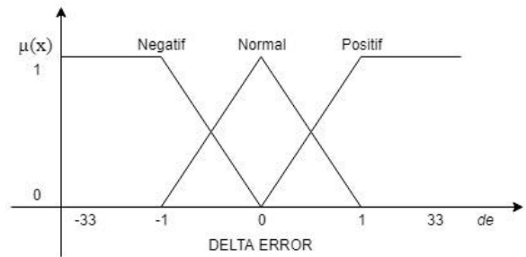
Gambar 11. Himpunan Fuzzy Error dan Delta Error Suhu
