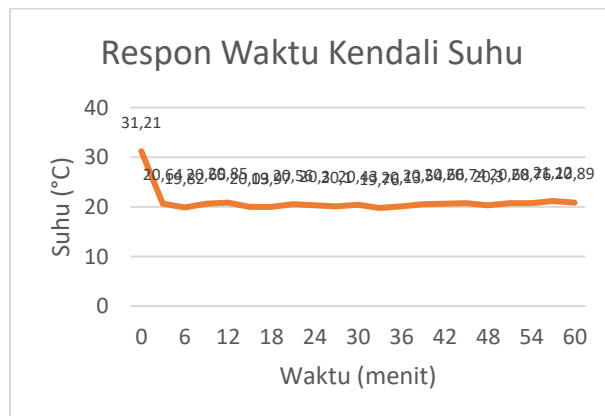
Gambar 17. Respon Waktu Kendali Suhu
