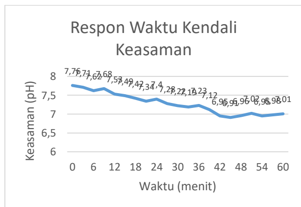
Gambar 16. Respon Waktu Kendali Keasaman
