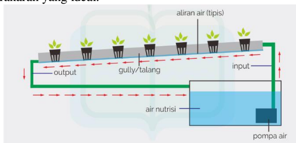
Gambar 2 Skema Sistem Hidroponik NFT (Sumber : Hidroponikpedia.com).
