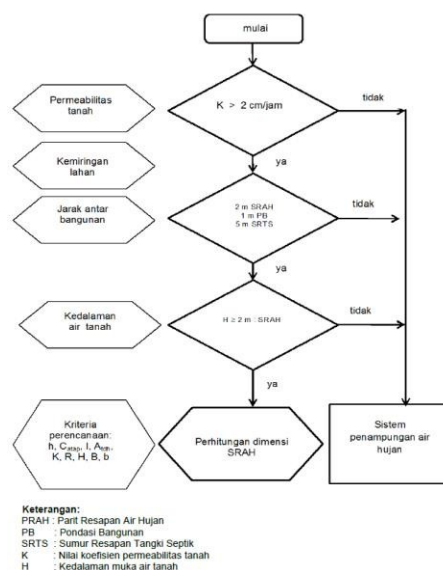
Gambar 2.2. Diagram Alir Langkah-Langkah Perencanaan Sumur Resapan
