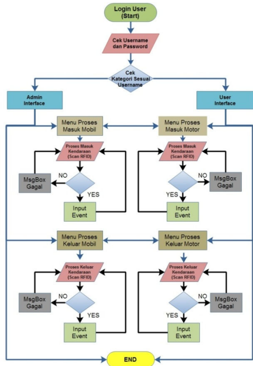
Gambar 5. Flowchart Sistem Manajemen Parkir Secara Umum
