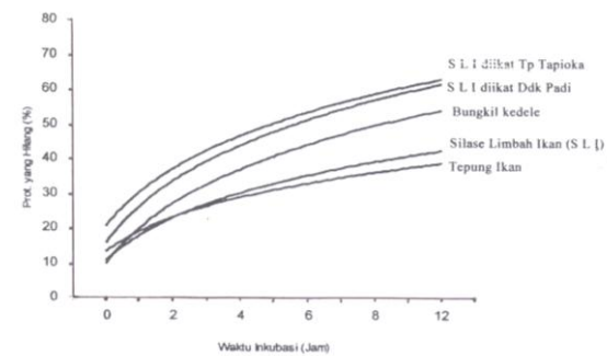
Gambar 1. Perbedaan pola degradasi protein dalam kantong nilon dari tepung ikan ( y = 14,07\ln(x) + 13,24 ; R^2 = 0,88 ), silase limbah ikan ( y = 17,58 \ln(x) + 10,55 ; R^2 = 0,96 ) bungkil kedele ( y = 24,43\ln(x) + 9,99 ; R^2 = 0,98 ), silase limbah ikan yang diikat dengan dedak padi ( y = 25,39\ln(x) + 15,81 ; R^2 = 0,94 ), dan silase limbah ikan yang diikat dengan tepung tapioka ( y = 25,39\ln(x) + 15,81 ; R^2 = 0,94 ).
