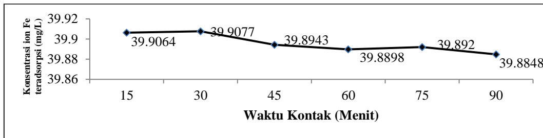
Gambar 4. Grafik Waktu Kontak Adsorben setelah aktivasi terhadap Fe^{2+}
