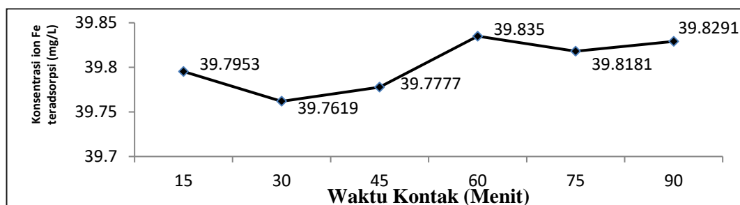
Gambar 3. Grafik Waktu Kontak Adsorben sebelum aktivasi terhadap Fe 2+
