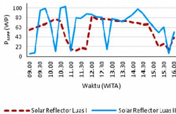
Gambar 5. Perbandingan luasan solar reflector terhadap titik daya maksimum ( P_{MPP} ) pada kecepatan angin ( v ) 4 m/s.
