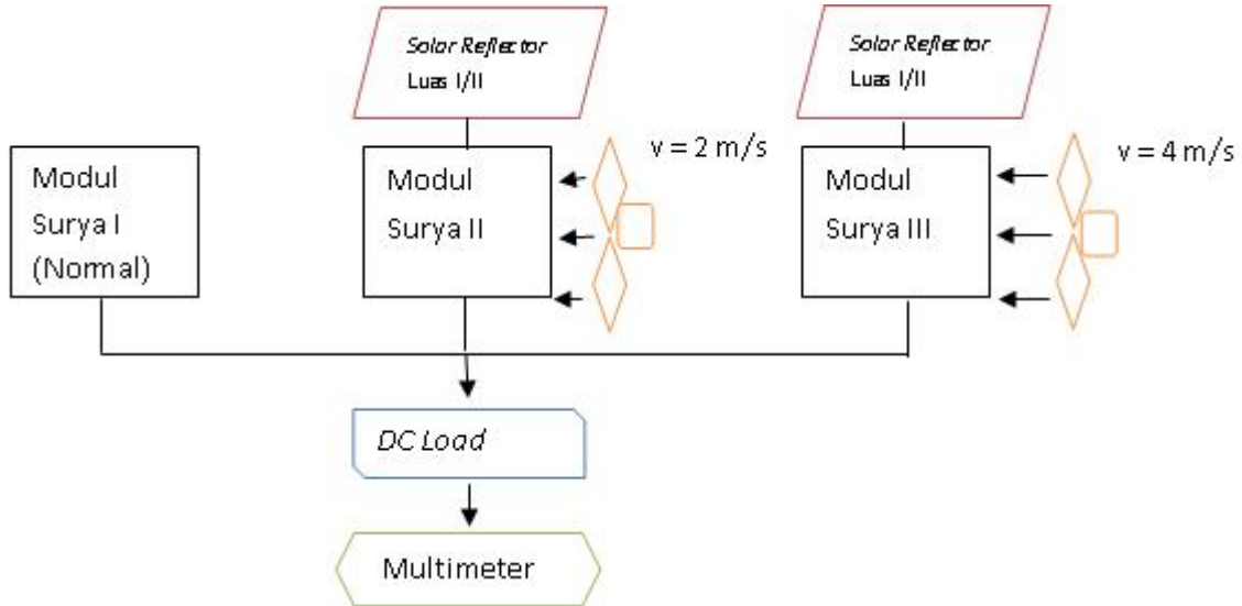
Gambar 1. Skema pengujian modul surya pada kondisi normal dan dengan perlakuan
