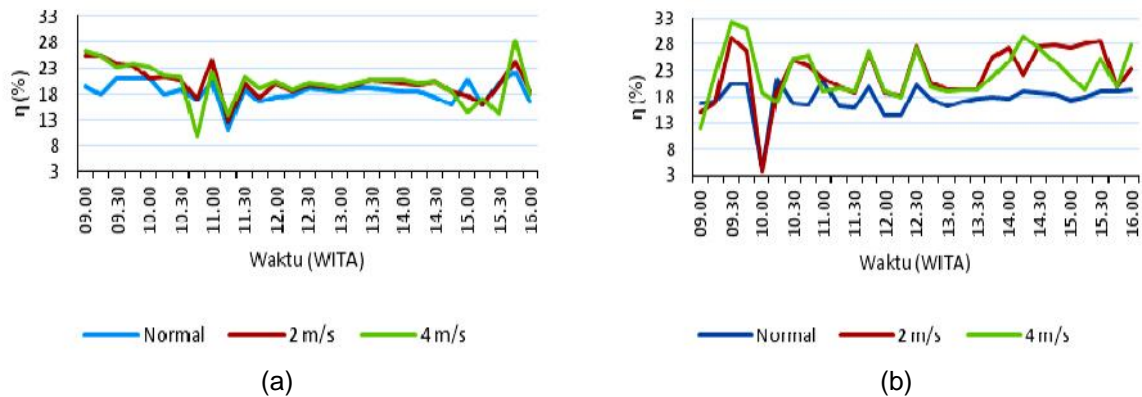
Gambar 6. Perbandingan efisiensi keluaran maksimum ( \eta ) untuk masing-masing variabel pada penggunaan solar reflector ; (a) luas I , dan (b) luas II.
