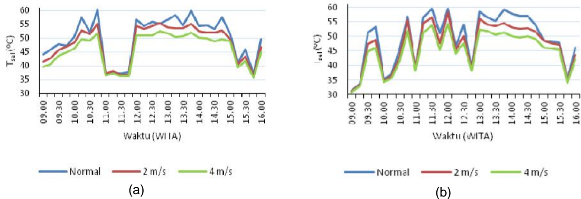
Gambar 2. Perbandingan temperatur sel surya ( T_{sel} ) untuk masing-masing variabel pada penggunaan solar reflector , (a) luas I, dan (b) luas II.
