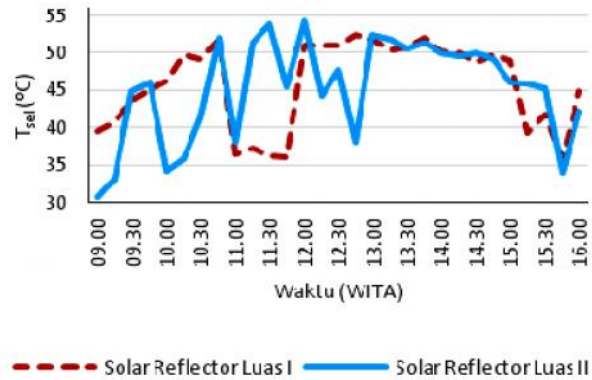
Gambar 3. Perbandingan luasan solar reflector terhadap temperatur sel surya ( T_{sel} ) pada kecepatan angin ( v ) 4 m/s.
