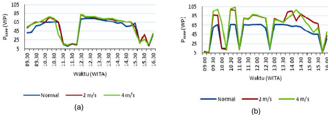
Gambar 4. Perbandingan titik daya maksimum ( P_{MPP} ) untuk masing-masing variabel pada penggunaan solar reflector, (a) luas I, dan (b) luas II.
