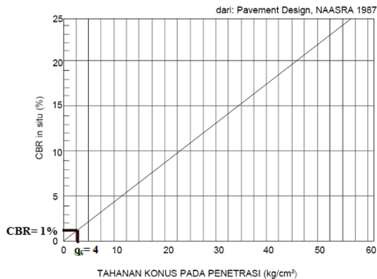
Gambar 2. Korelasi Nilai CBR dan Konus
