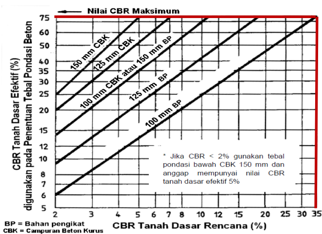
Gambar 3. Grafik CBR Efektif dan Tebal Pondasi Bawah
