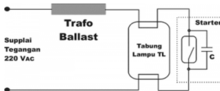
Gambar 7. Rangkaian Lampu TL Dengan Trafo Ballast [3].
