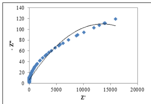
Gambar 4. (a) Grafik Nyquist Sampel CNTs/LiCl, (b) Perbesaran dari Grafik Nyquist Sampel CNTs/LiCl 15%
