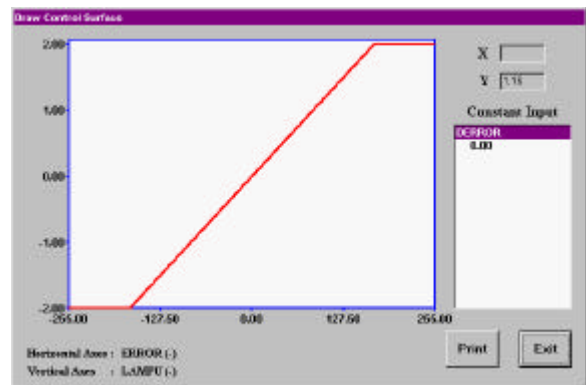
Gambar 10. Grafik Output Lampu terhadap Input Error dengan \Delta\_Error = 0
