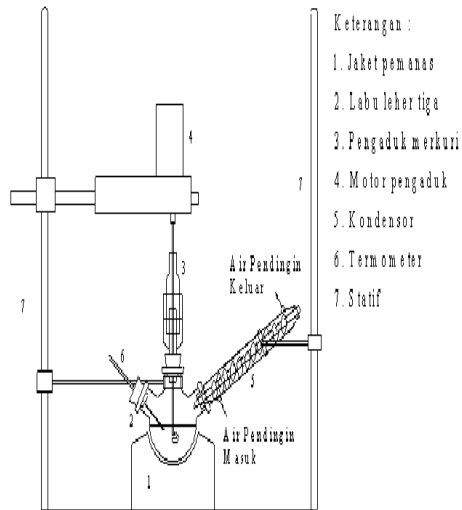
Gambar 4. Rangkaian Alat Pemasak Alang-Alang
