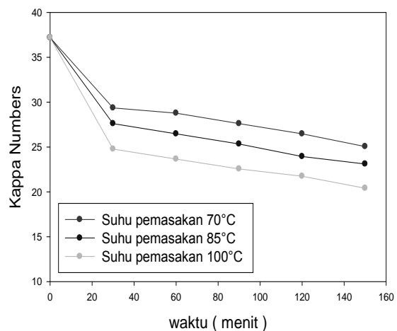
Gambar 10. Hubungan Antara Waktu Terhadap Bilangan Kappa Untuk Berbagai Suhu Pada Konsentrasi Asam Asetat 90%
