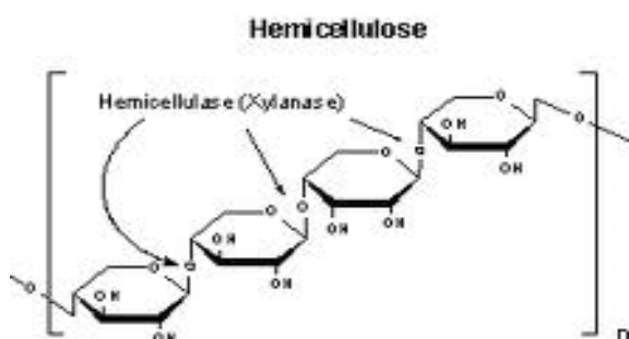
Gambar 3. Senyawa Hemiselulosa [14]
