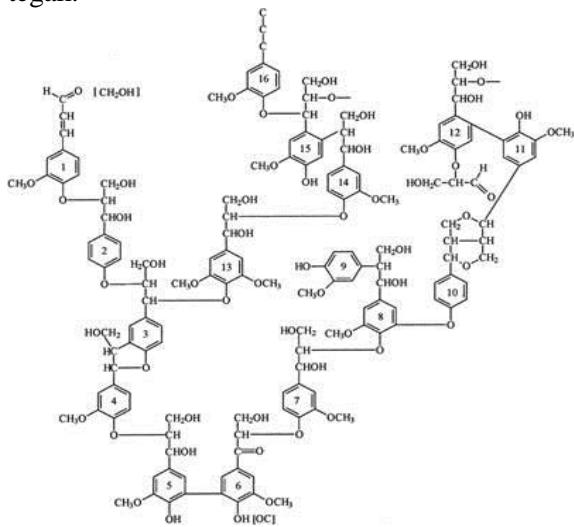
Gambar 2. Struktur Lignin [15]
