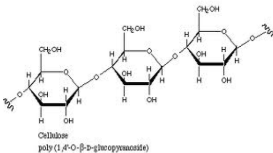
Gambar 1. Rumus Molekul Selulosa
