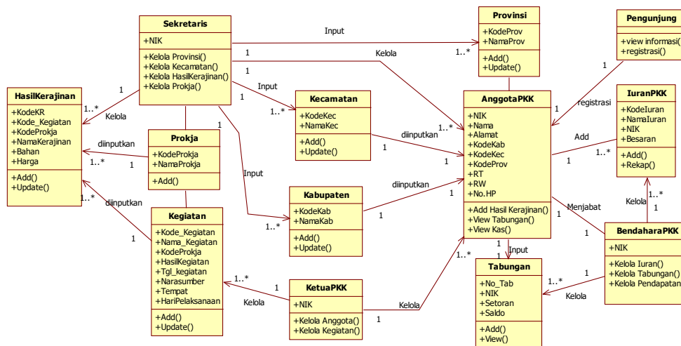
Gambar 2. Diagram Kelas Sistem Pengelolaan Kegiatan Pemberdayaan Kesejahteraan Keluarga di Universitas Muria Kudus Berbasis Web
