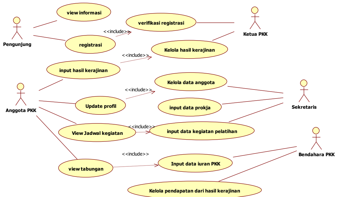
Gambar 1. Diagram Use Case Sistem Pengelolaan Kegiatan Pemberdayaan Kesejahteraan Keluarga Di Universitas Muria Kudus Berbasis Web
