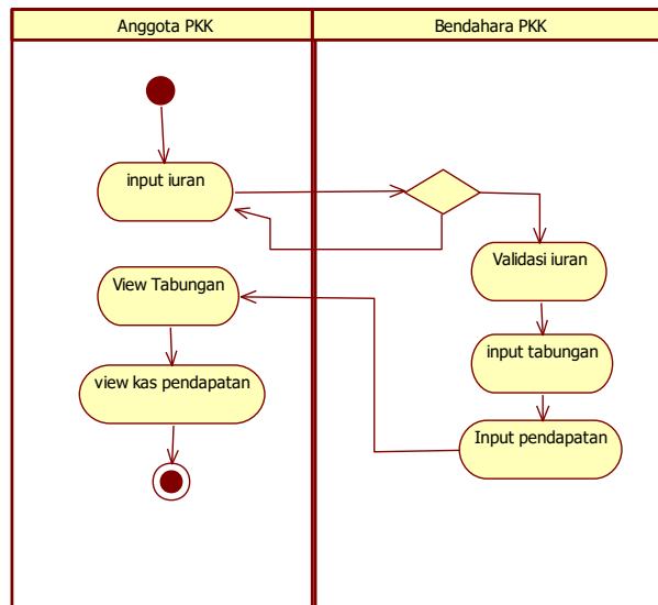
Gambar 6. Diagram Aktifitas Iuran PKK Sistem Pengelolaan Kegiatan Pemberdayaan Kesejahteraan Keluarga di Universitas Muria Kudus Berbasis Web
