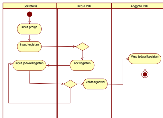
Gambar 5. Diagram Aktifitas Kelola Kegiatan Sistem Pengelolaan Kegiatan Pemberdayaan Kesejahteraan Keluarga Di Universitas Muria Kudus Berbasis Web
